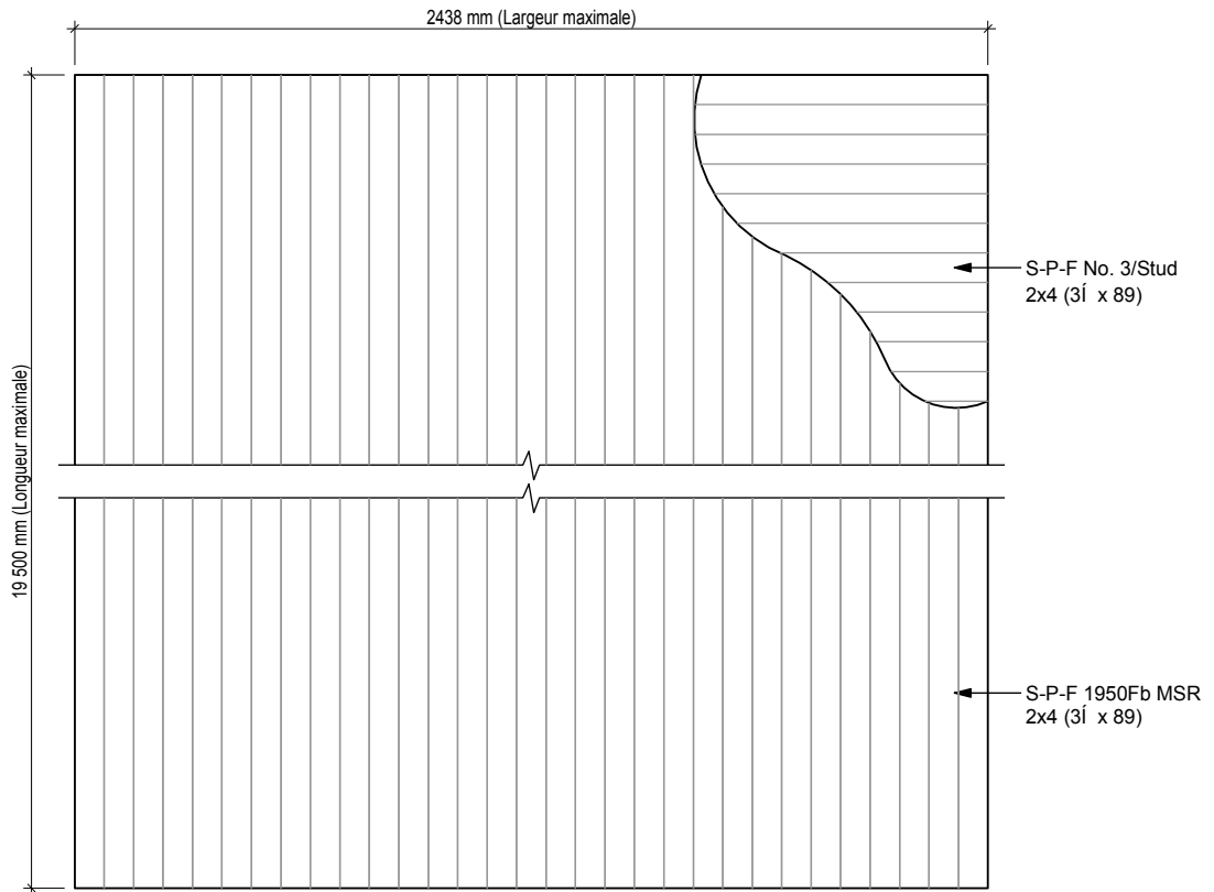
A ÉLÉVATION - ÉCH.: 1: 25
