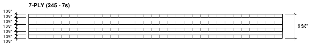
B SECTION ÉCH.: 1: 25
