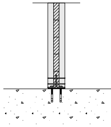
D2 BASE POINT SOLE PLATE
