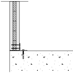
D1 BASE POINT SOLE BRACKETS
